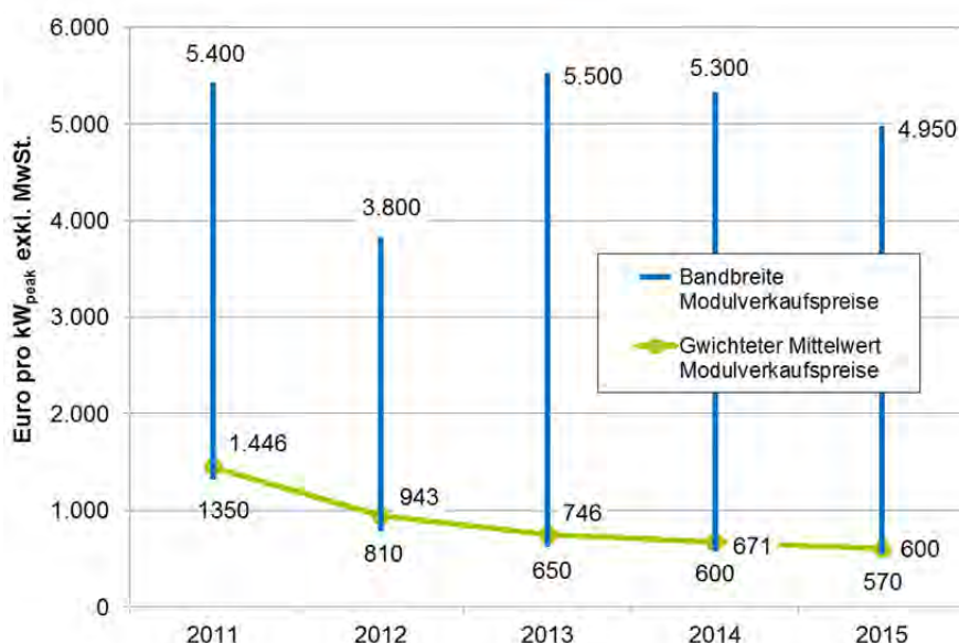
Abbildung 7.6: Gewichteter Mittelwert und Bandbreite der Modulverkaufspreise der österreichischen Modulhersteller 2011 bis 2015, Werte exkl. MwSt.; Anzahl der Nennungen: 2011: n=6, 2012: n=5, 2013: n=7, 2014: n=5, 2015: n=4; Quelle: Erhebung Technikum Wien.
