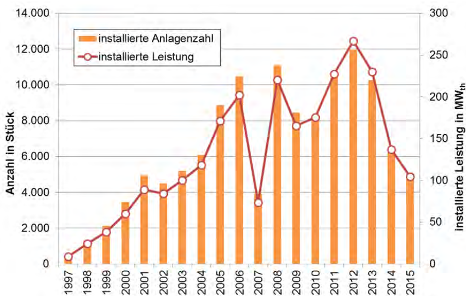
Abbildung 6.3: Jährlich installierte Pelletsboiler < 100 kW th in Stück. Quelle: LK NÖ (2016a)
